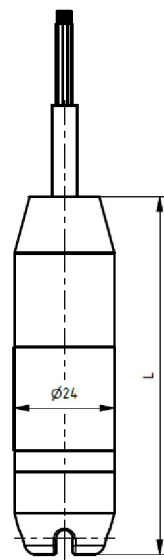
Fig. 9 Offene Ausführung
