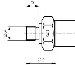
Fig. 5 - G 1/4 A
