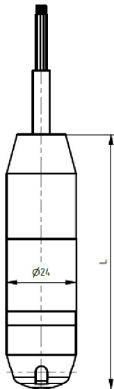
Fig. 8 Geschlossene Ausführung
