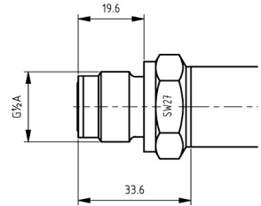
Fig. 4 - G 1/2 A, Membrane frontbündig
