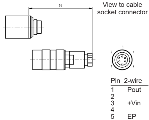
Fig. 13 - Binder 723, 5 pins
